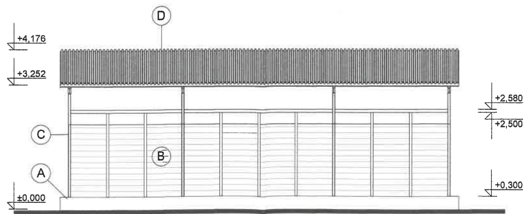
SO 10.2 Pohľad severozápadný
