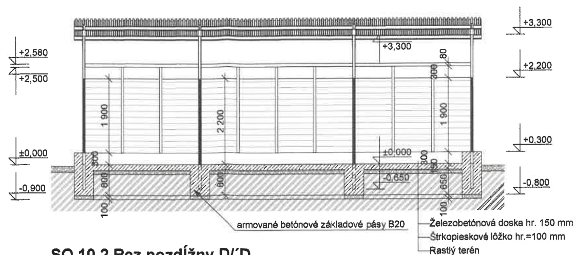
SO 10.2 Rez pozdĺžny D/D
