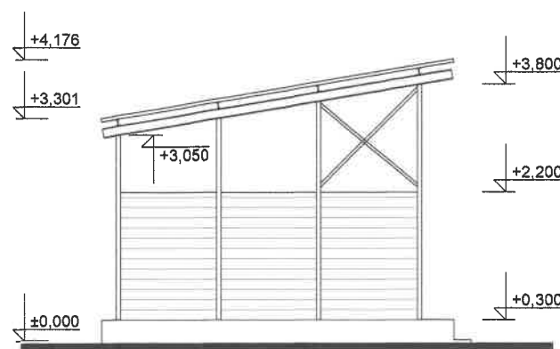
SO 10.2 Rez pozdĺžny D/D
