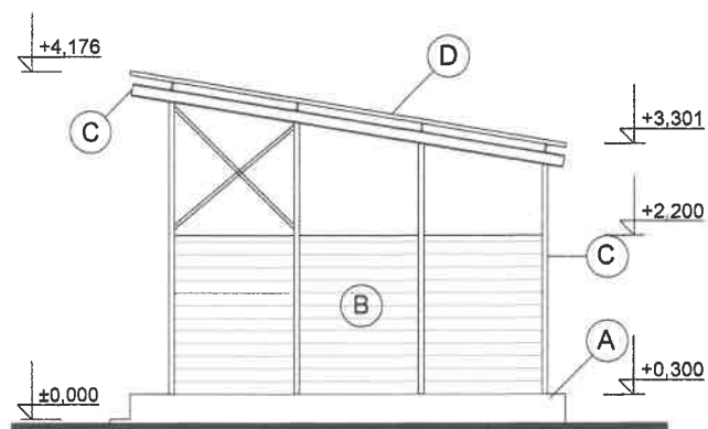
SO 10.2 Pohľad juhovýchodný
